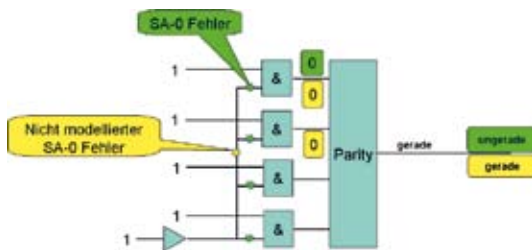
Abbildung 1.10: Problemstellung für einen Layout-basierten ATPG
