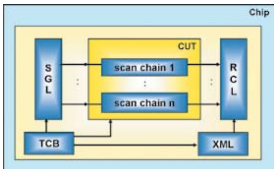
Abbildung 1.05: TK Logik mit Response-Compaction-Logik
